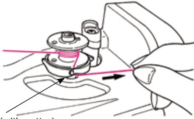
Guide (with cutter) Guía (con cortador) Guide (avec couteau) Guida (con tagliafilo)
