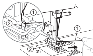
① Hilo superior ② Hilo inferior
