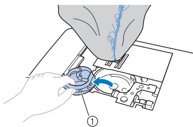
① Cestello della spolina
