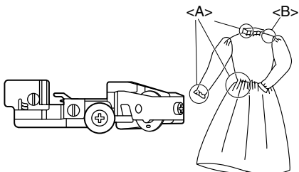
<A> Einsatz von Gummiband <B> Einsatz von Schrägband
