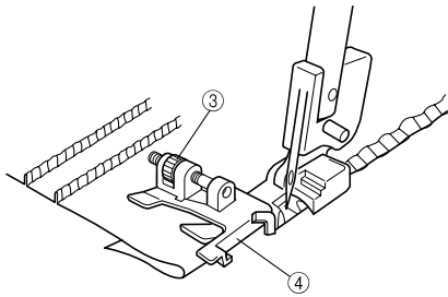
③ Stellschraube ④ Führung am Nähfuß
