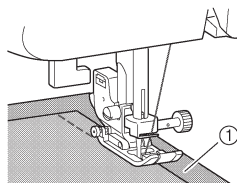
① Entretela ou papel
