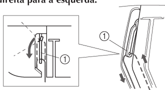
① Alavanca do puxa-fio
